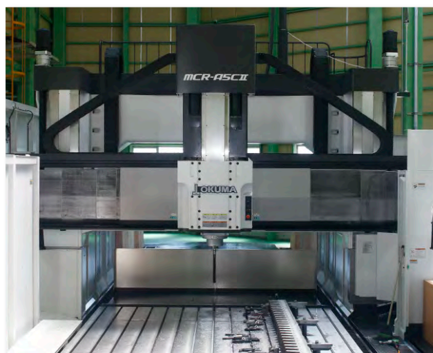
MCR-A5C II (35) / オークマ株式会社 テーブル: 3500×6000mm
